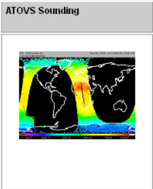
POES
